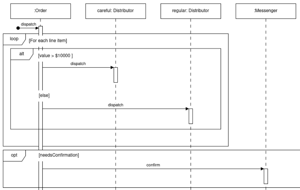
Figura 5.4: Esempio sequence diagram
